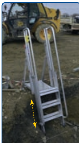
Piètements télescopiques réglables sur 4 hauteurs.
